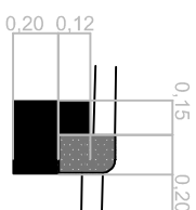
KRAWEŹNIK NA JAZDOWY NA ŁAWIE BETONOWEJ
