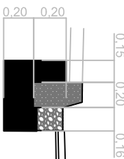
KRAWEŹNIK ZE ŚCIEKIEM NA ŁAWIE BETONOWEJ
