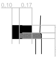
OBRZEŻE CHODNIKOWE NA ŁAWIE BETONOWEJ
