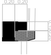
KRAWEŹNIK WYSTAJĄCY NA ŁAWIE BETONOWEJ
